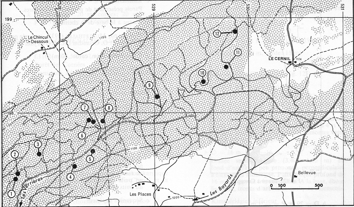
Fig. 122. Les gouffres de la forêt des Cornées (Les Bayards - Les Verrières).
